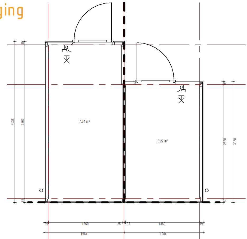
plattegrond
