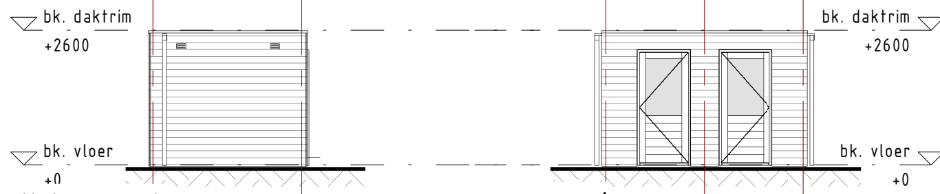
linkergevel
