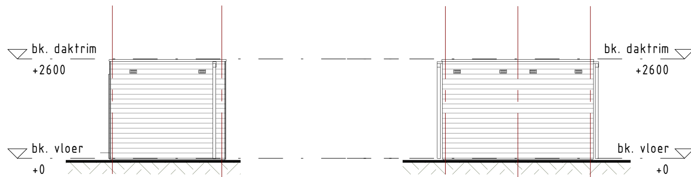
rechtergevel
